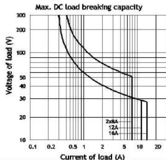
Gleichstrom - Lastgrenzkurve
