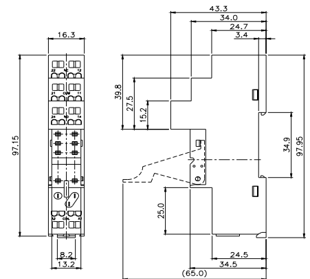
Module, Haltebügel
